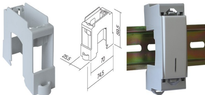
1M ADAPTER DIN sínre
