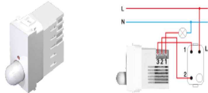
FORGATÓGOMBOS VÁLTÓ DIMMER 40-300W
