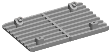
MA 65 összekötő elem
