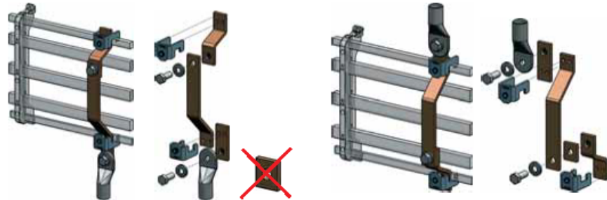
Csatlakozás alulról
