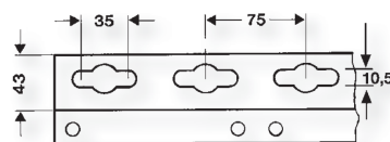
Rögzítő raszterek szerelősínekhez
