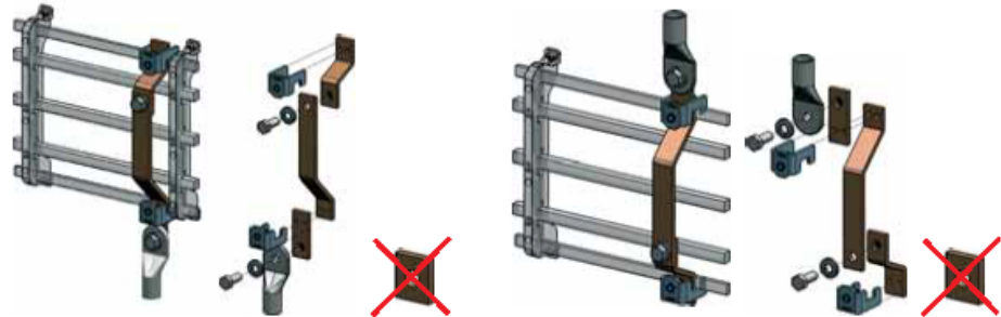
Csatlakozás alulról
