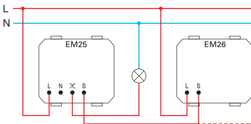
(1) két vezetékes csatlakozás two-wire connection
