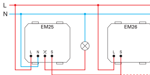
(2) három vezetékes csatlakozás three-wire connection
